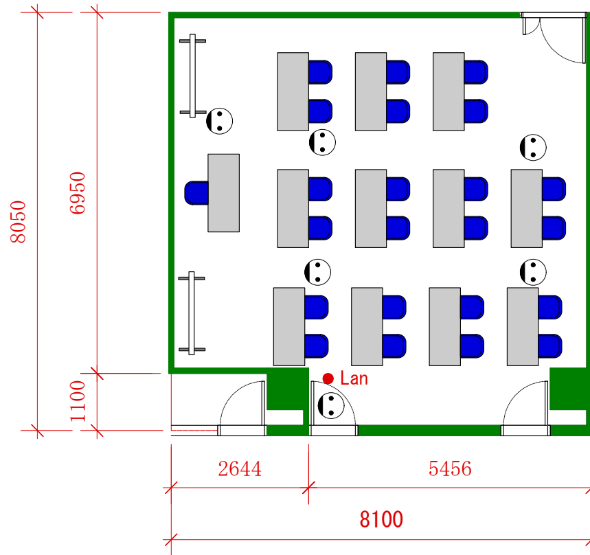
3階小会議室 57.7㎡
